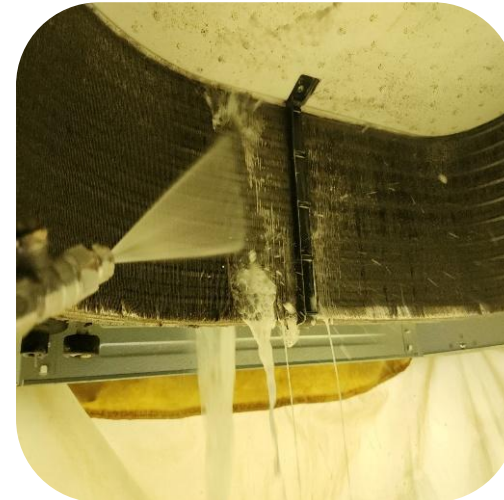
고압 세척
