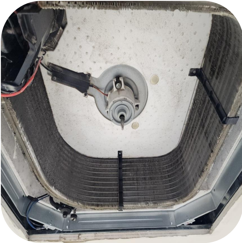
세척 전
